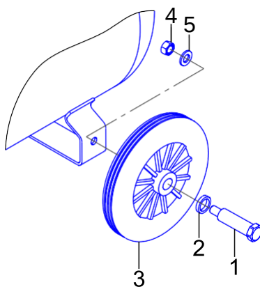
1 - Болт
