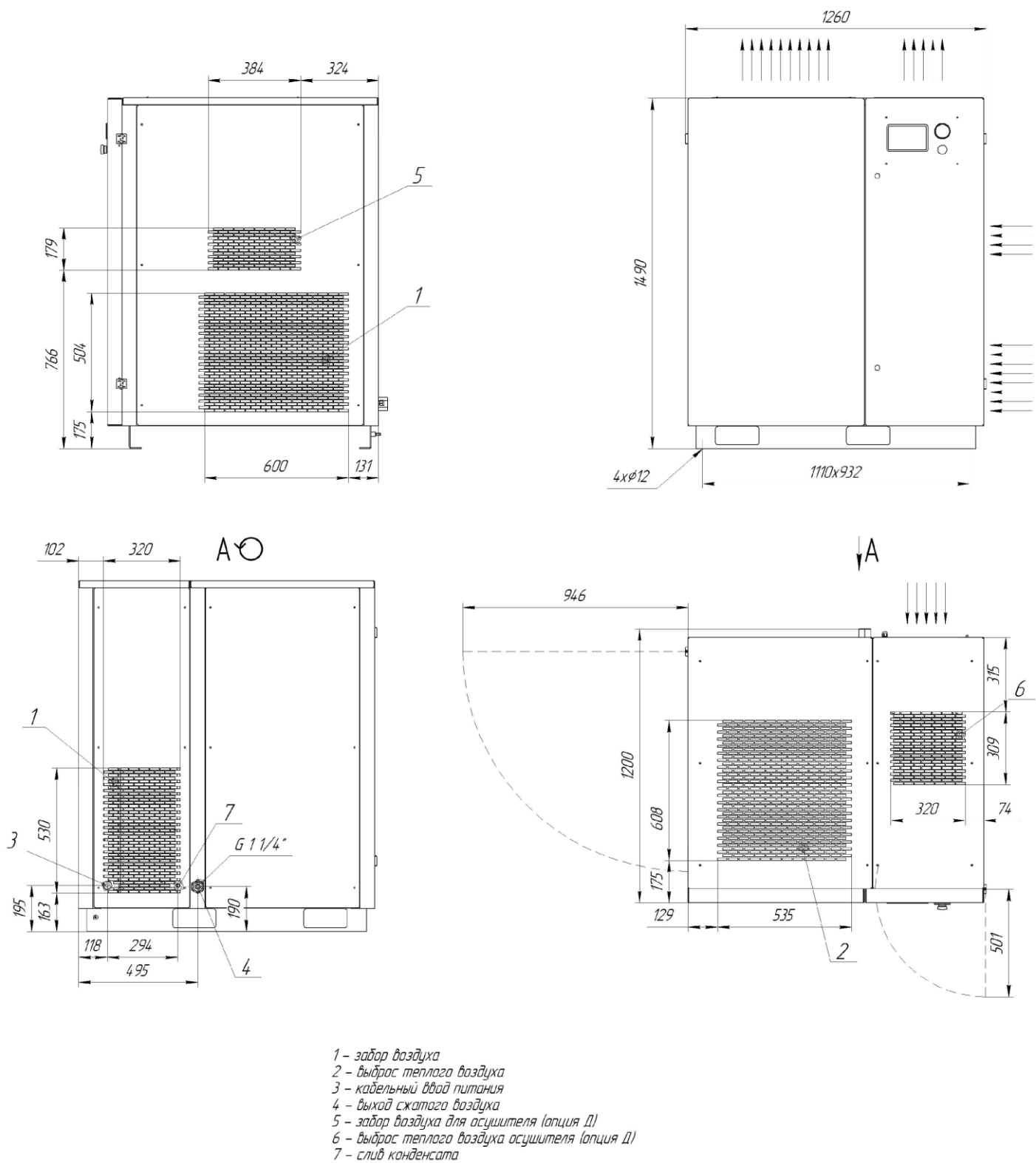
Рис.8 Присоединительные и установочные размеры компрессорной установки
